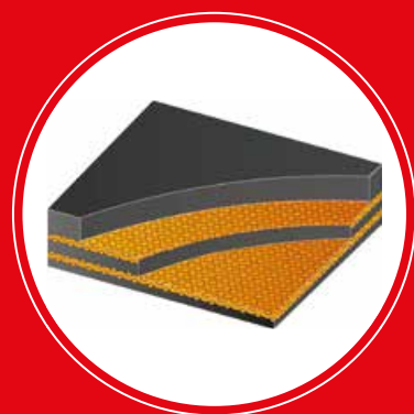
DUNLOFLEX COUPE TRANSVERSALE
