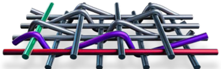
Die einzigartige gerade Kettfädenbeschaffenheit der UsFlex-Karkasse
